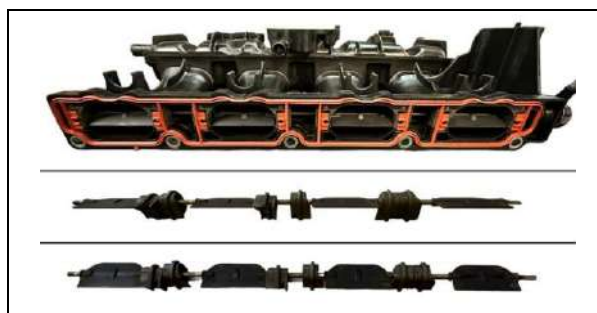
3AD) Volet dans le collecteur d'admission Flap in the intake manifold
